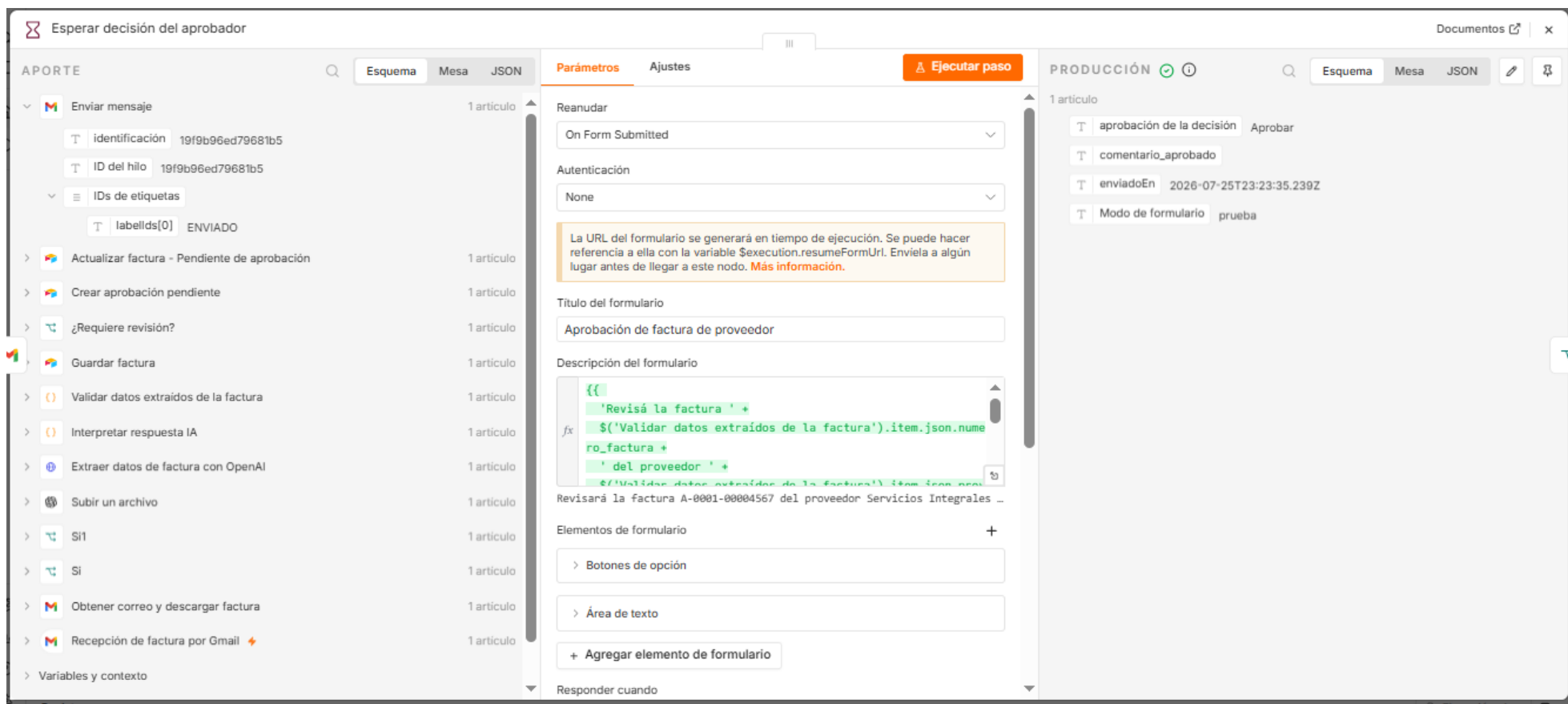
Figura 6. Punto de espera y decisión Human-in-the-Loop.
